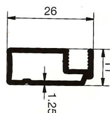
PROFILO TELAIO FISSO
